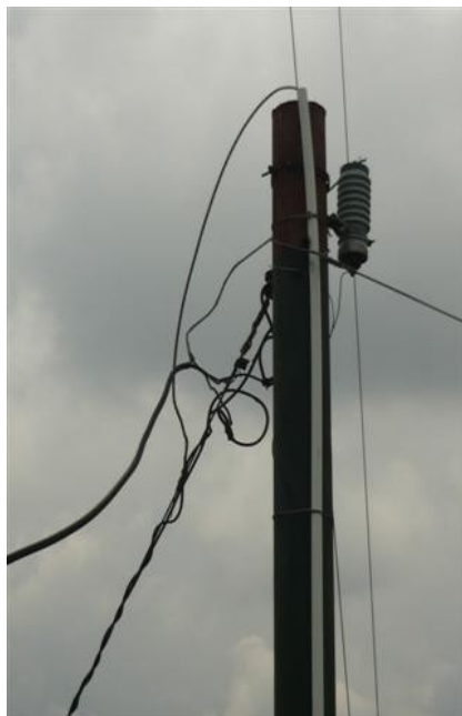
Acometida eléctrica
