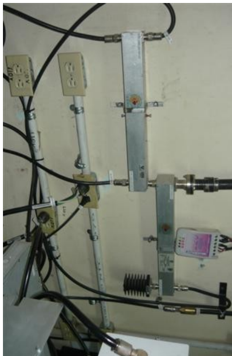
Diplexado canal 7 y 11
