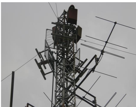
Antenas existentes
