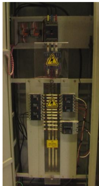
acometida eléctrica
