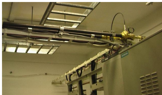
escalerilla interna
