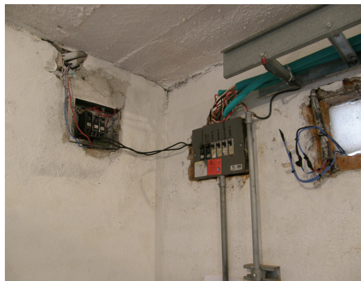
Acometida eléctrica
