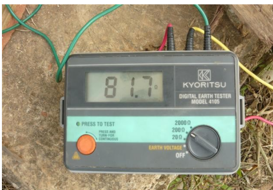
Medición tierra antena satelital
