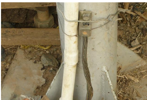
Sistema de puesta a tierra antena satelital
