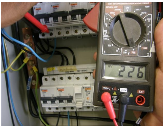
MEDIDAS DE VOLTAJE Y CORRIENTES
