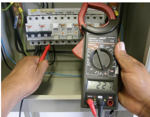
MEDIDAS DE VOLTAJE
