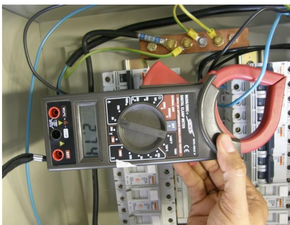
MEDIDAS DE VOLTAJE Y CORRIENTES
