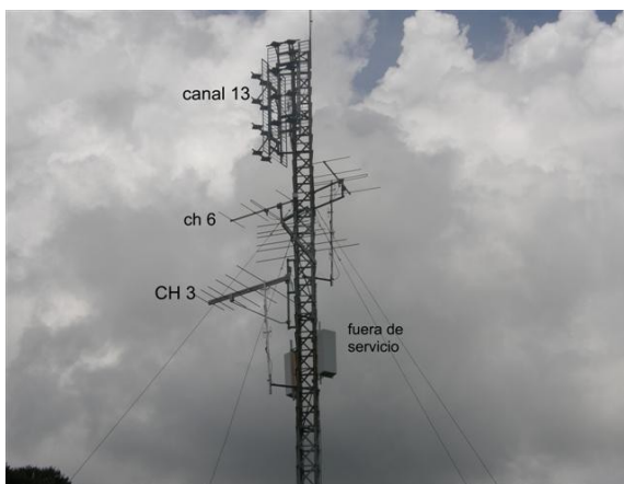
Antenas existentes
