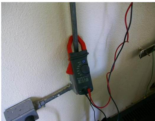
Medida Fase - T
