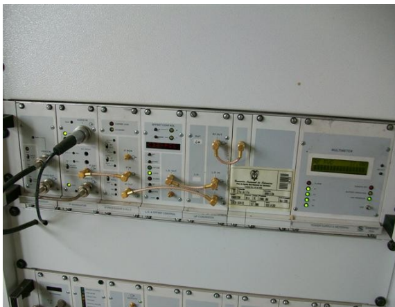
Transmisor C1
