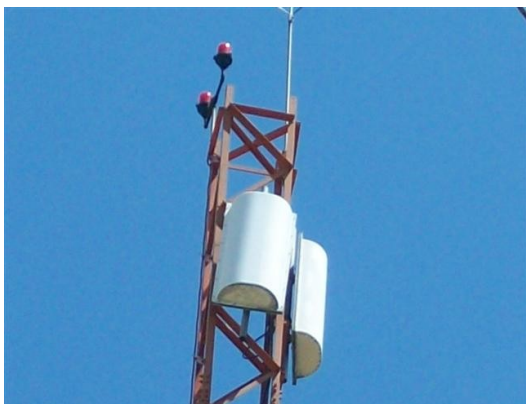
Sistema de antenas C1, SC y SI. (Triplexados)
