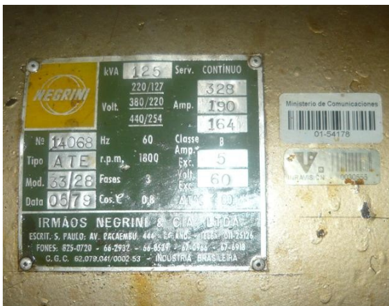
Detalle placa de información
