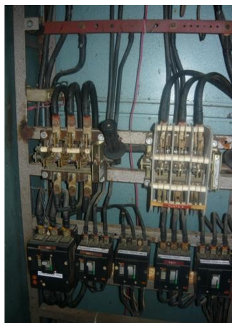
Acometida Eléctrica
