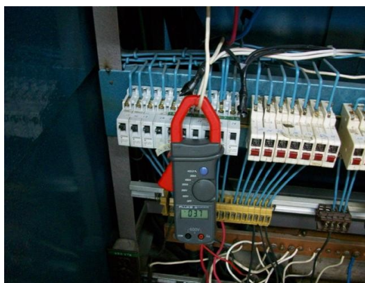
Medida Corriente Mincomunicaciones
