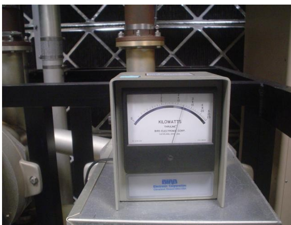
Medida Potencia Transmisor Principal Canal
