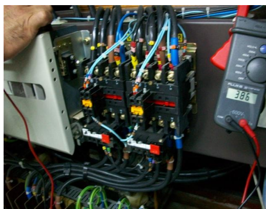
Medida Tensión S-T
