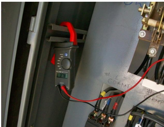
Tensión R-S
