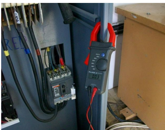
Tensión N-T
