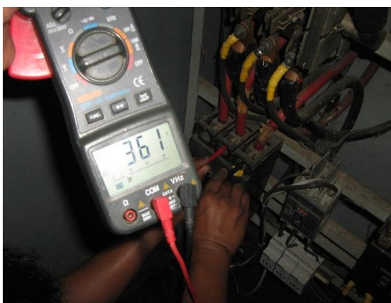
Medición de voltaje Fases S' - T'
