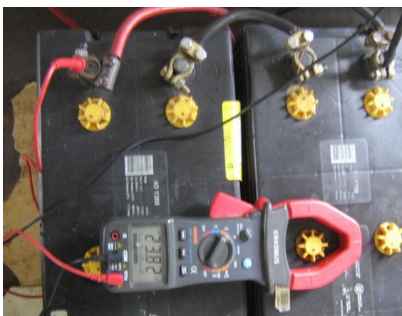
medición de baterías planta Perkins
