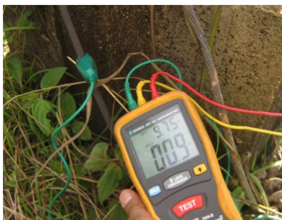
Medición sistema de tierra pararrayos
