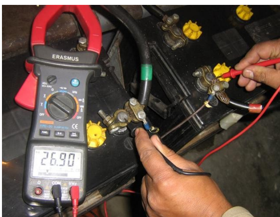
Medida baterías planta eléctrica
