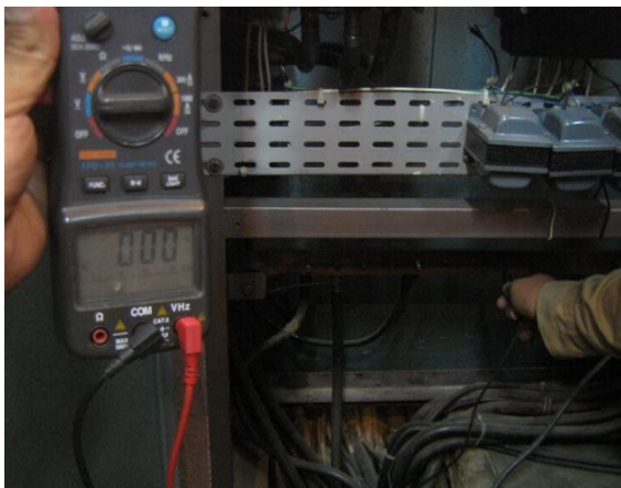
Medición de Volt N- T
