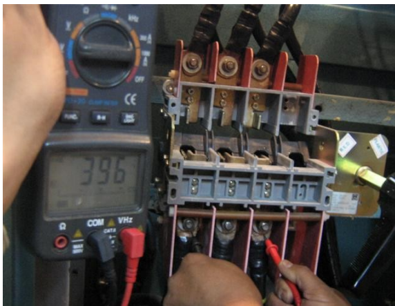
Medición de Volt Fase R - T
