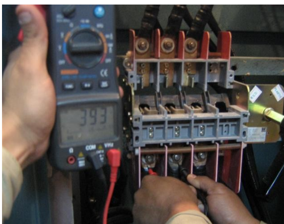
Medición Volt fases R - S
