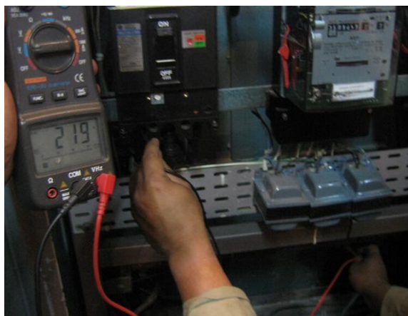
Fase R - N
