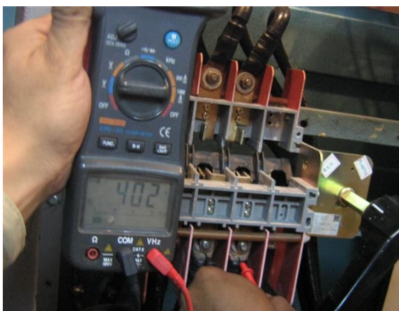
Medición volt fases S- T
