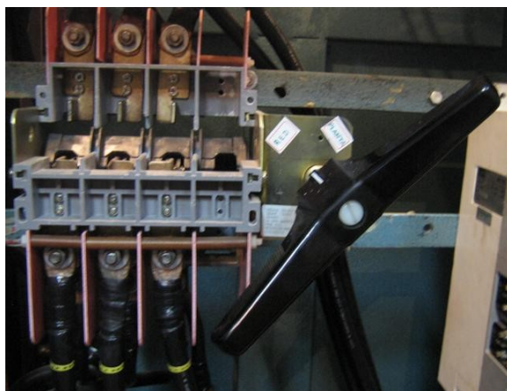
Transferencia manual red - planta
