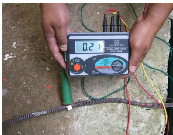
Medidas de sistema pararrayos torre
