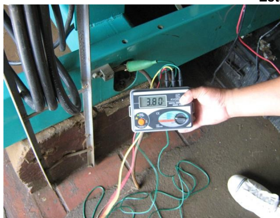
Medición de tierra salón de plantas
