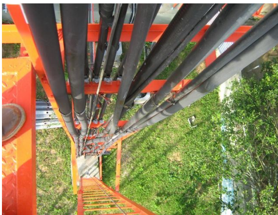
Lineas de transmisión 2
