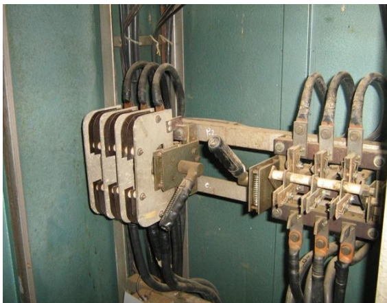
Transferencia Red - Planta Estación
