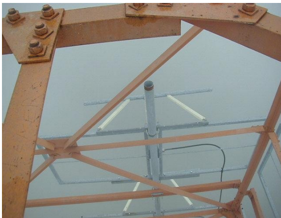
Antena
