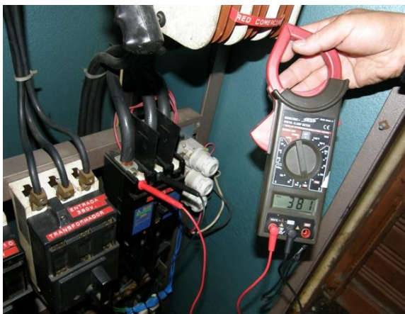
Medida de voltaje en rack principal)
