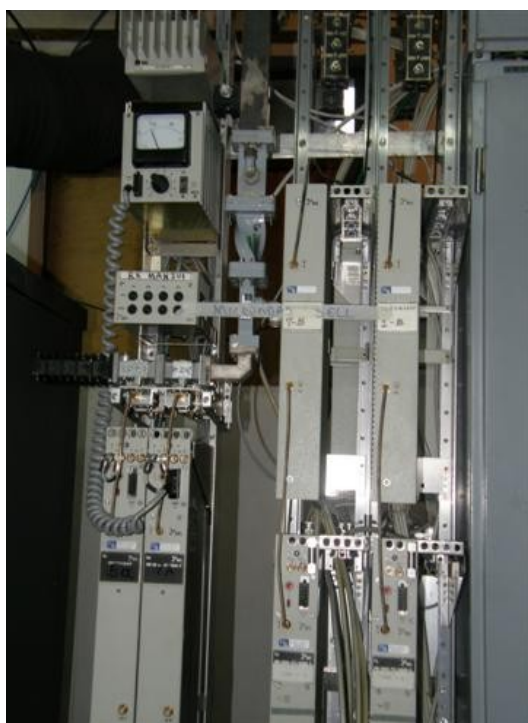
microondas alcatel seel
