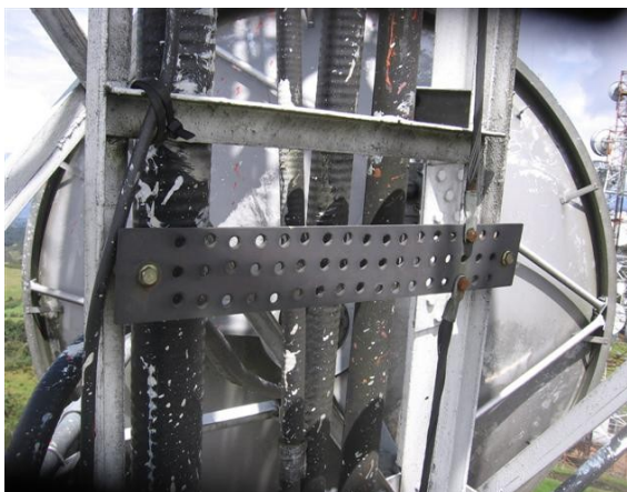
Platina de tierra en torre
