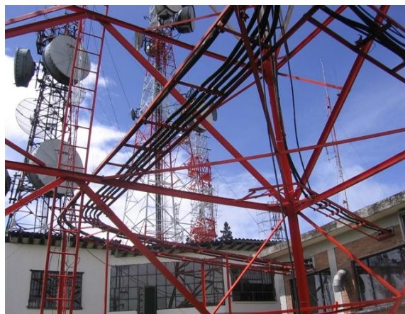
Vista escaleras horizontales
