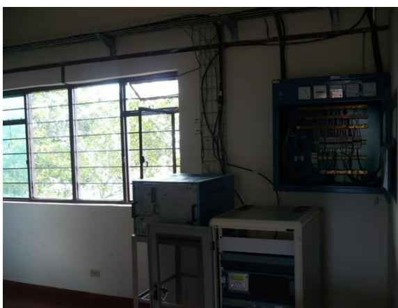
Transmisor FM, Transmisor TRO, Tablero totalizador
