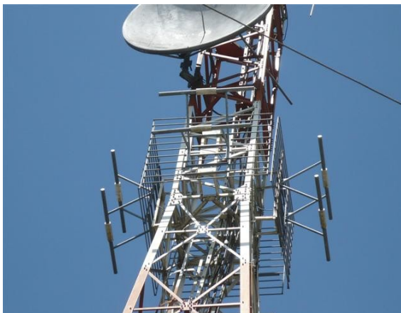
Antenas FM Fig.2
