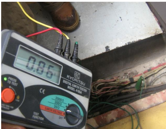
Medición tierra salón de equipos
