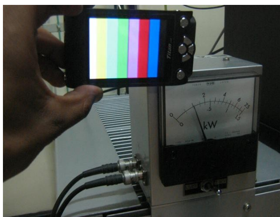
Medición de potencia Tx NEC S - C
